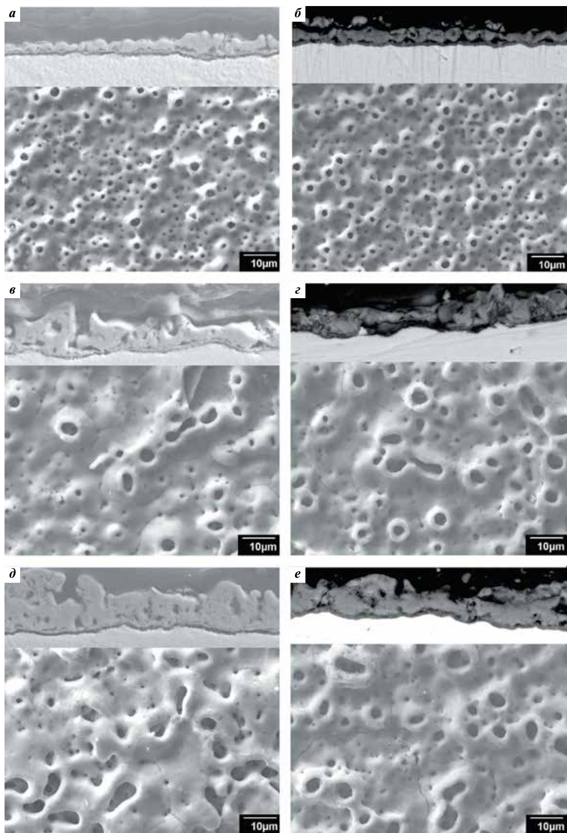
Рис. 2. Изображения покрытий методом плазменно-электролитического оксидирования: а, в, д — крупнозернистое покрытие сплава; б, г, е — ультрамелкозернистое покрытие сплава, полученных при различном напряжении: а, б — 385 В; в, г — 450 В; д, е — 480 В
