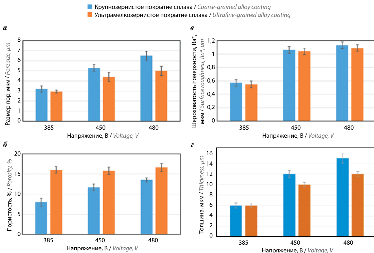
Рис. 3. Влияние напряжения на параметры покрытия методом плазменно-электролитического оксидирования: а – размер пор; б – пористость; в – шероховатость поверхности; г – толщина покрытий.
