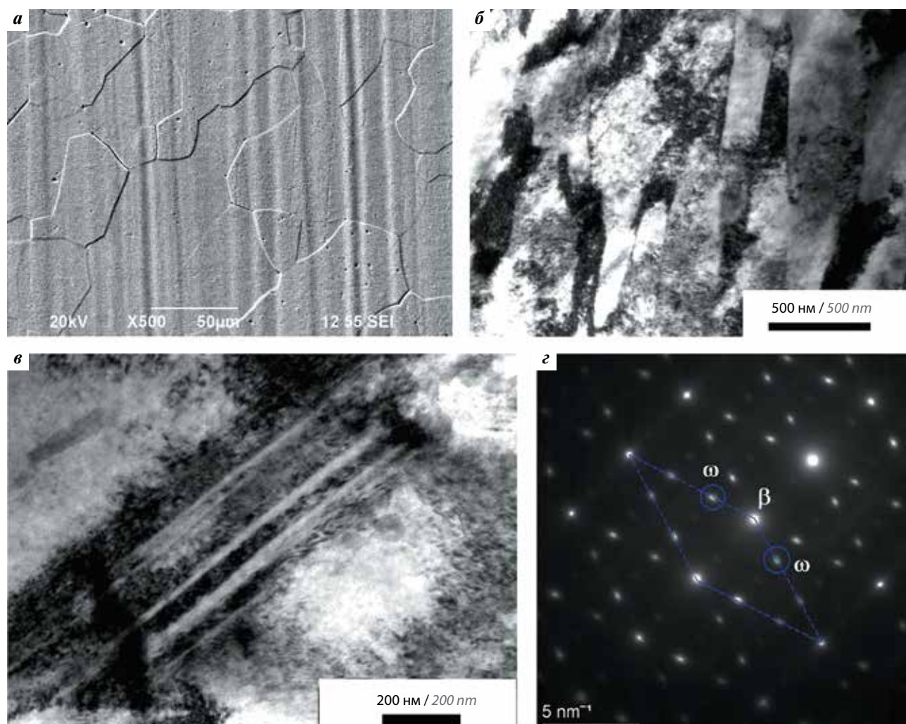
Рис. 1. Структура сплава: а – в крупнозернистом состоянии; б – в ультрамелкозернистом состоянии; в – изображение микродвойников; г – картина микродифракции ультрамелкозернистого сплава
